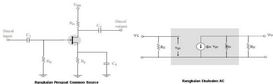
Gambar 2. 13 Rangkaian penguat
