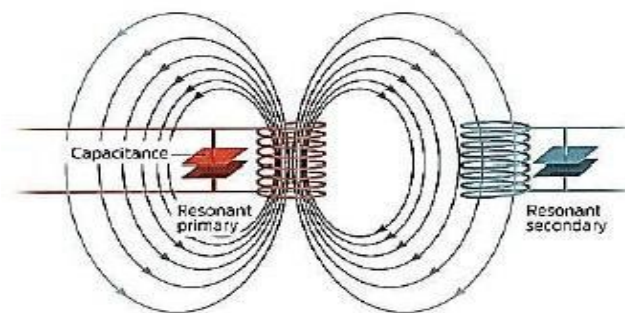
Gambar 2. 7 Resonansi Kopling Induktif
