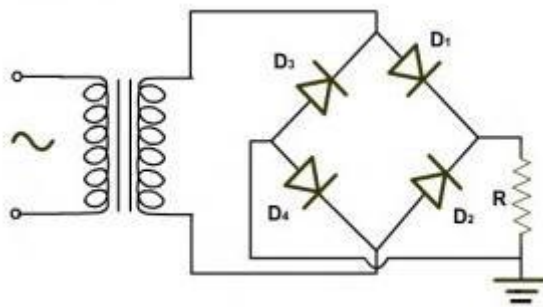
Gambar 2.21 Rangkaian Penyearah Gelombang Penuh
