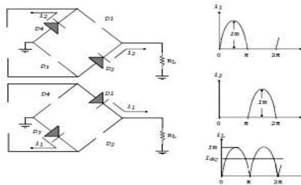
Gambar 2.11 Proses Penyearah Gelombang Penuh
