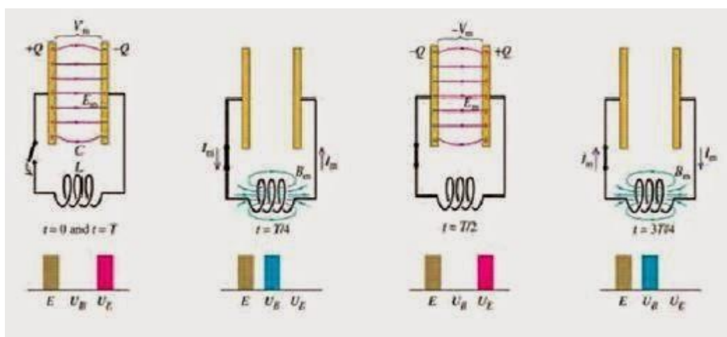
Gambar 2.18 Prinsip Kerja Rangkaian LC
