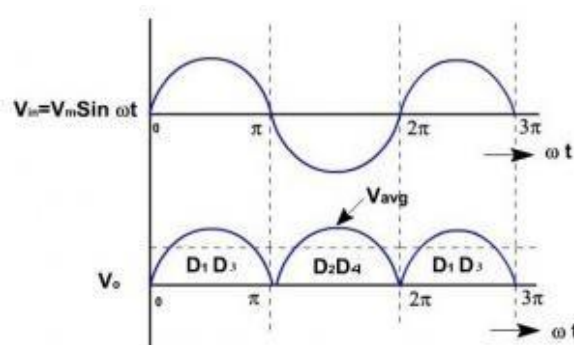
Gambar 2.22 Grafik Sinyal Rangkaian Penyearah Gelombang Penuh
