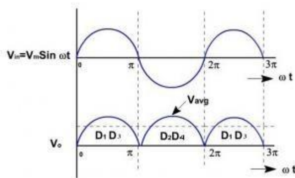
Gambar 2.10 Bentuk Sinyal Hasil Penyearah Gelombang Penuh
