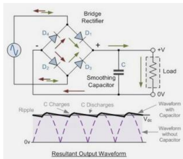
Gambar 2.12 Penyearah Dilengkapi Filter Kapasitor
