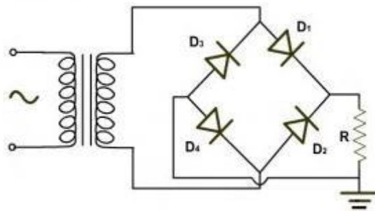
Gambar 2.9 Penyearah Gelombang Penuh
