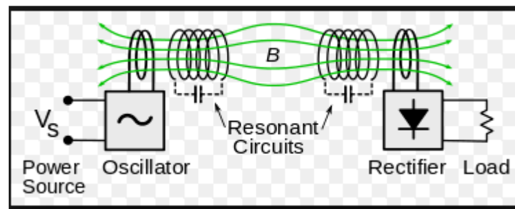
Gambar 2. 3 Skema sederhana transfer energi wireless dengan prinsip resonansi elektromagnetik
