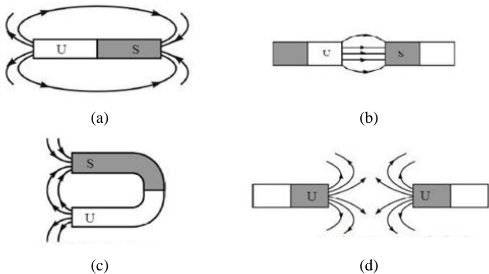
Gambar 2. 4 (a) Arah garis gaya magnet batang, (b) Arah garis gaya dua kutub magnet yang tidak sejenis, (c) Arah garis-garis gaya magnet U, (d) Arah garis gaya dua kutub magnet yang sejenis.
