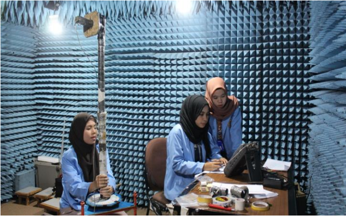
Pengukuran Polaradiasi dan Gain Antena
