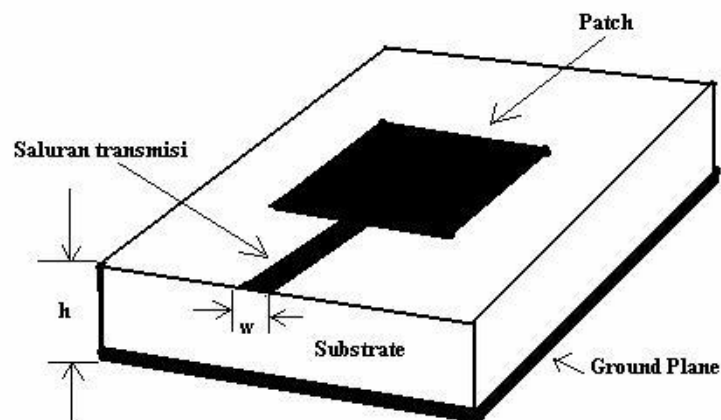
Gambar 2.5 Bentuk umum antena microstrip [3].
