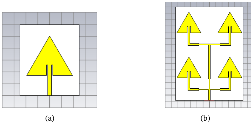
Gambar. 2.10 Struktur Antena Mikrostrip, (a) Antena Mikrostrip Patch Tunggal, (b) Antena Mikrostrip Array 4 Elemen.
