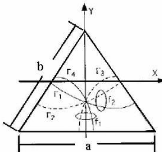
Gambar. 2.9 Antena Mikrostrip Patch Segitiga [13].
