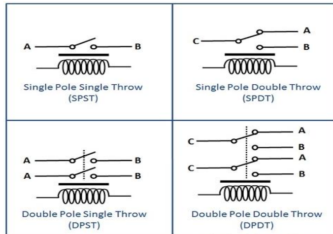
Gambar 2.3. Jenis Relay Berdasarkan Jumlah Pole dan Throw [4][3]
