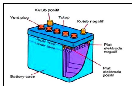
Gambar 2.7. Konstruksi Aki [10]
