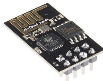
Gambar 2.22. ESP 8266 [20][2]
