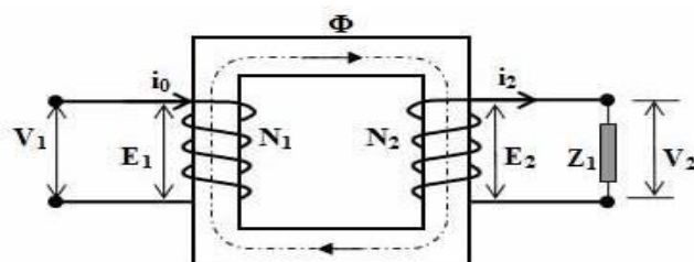
Gambar 2.9. Prinsip kerja Transformator [12][1]
