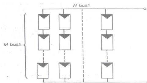
Gambar 2.19 Rangkaian seri-pararel PV
