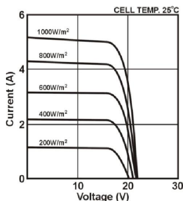
Gambar 2.21 Karakteristik Photovoltaic
