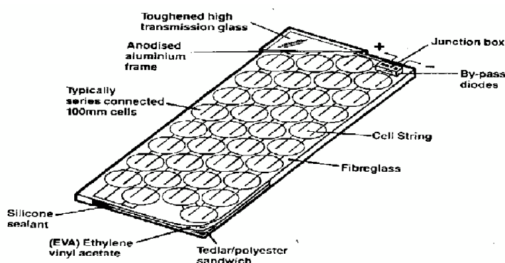
Gambar 2.18 Konfigurasi sebuah modul fotovoltaik.
