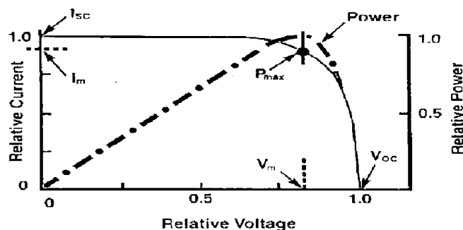
Gambar 2.20 Kurva Arus-Tegangan Dari Sebuah Modul Surya
