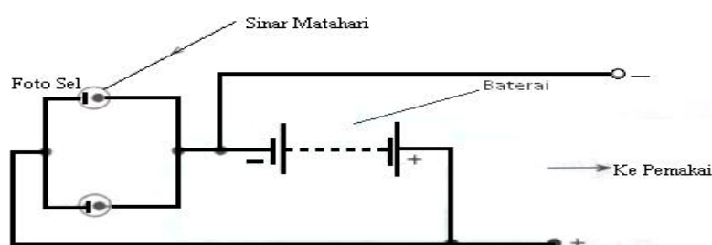
Gambar 2.1 Foto sel dan baterai aki (B) sebagai sumber energi listrik
