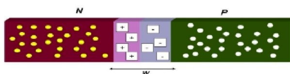
Gambar 2.6 : Semikonduktor Tipe-P dan Tipe-N Bersatu
