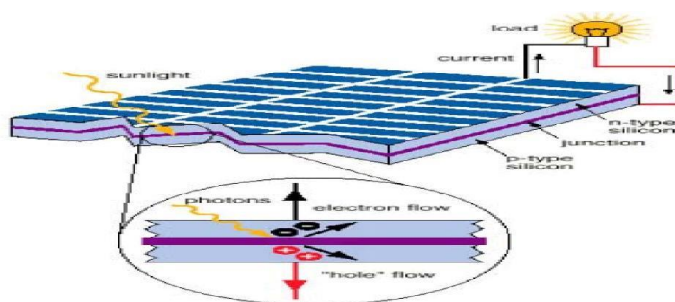
Gambar 2.3 Konversi cahaya matahari menjadi listrik
