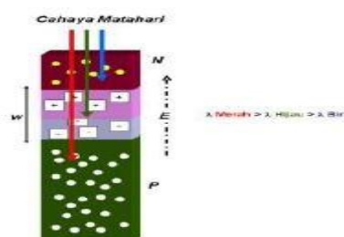
Gambar 2.8 : Konversi Cahaya Pada Semikonduktor P-N
