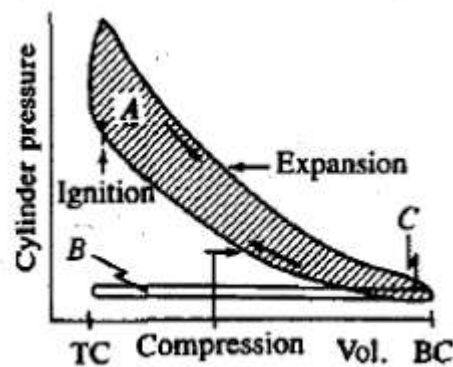
Gambar 2.2 Siklus Aktual Motor Diesel 4 Langkah (Cengel & Boles, 1994)
