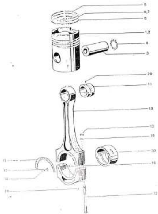
Gambar 2.17 Rangkaian Piston
