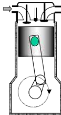
Gambar 2.3 Langkah Hisap
