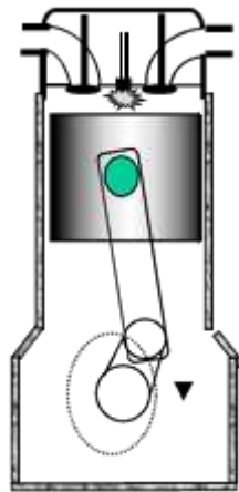
Gambar 2.5 Langkah Usaha
