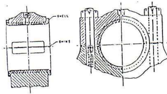
Gambar 2.22 Klasifikasi Bantalan
