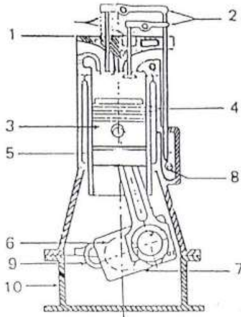
Gambar 2.10 Sketsa Mesin
