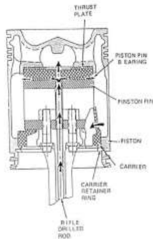
Gambar 2.16 Rangkaian Piston
