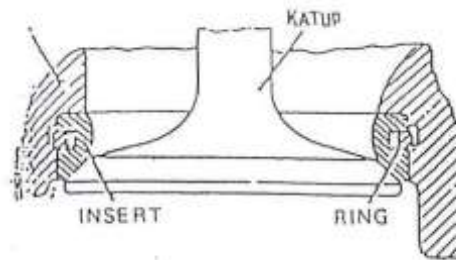
Gambar 2.15 Dudukan katup
