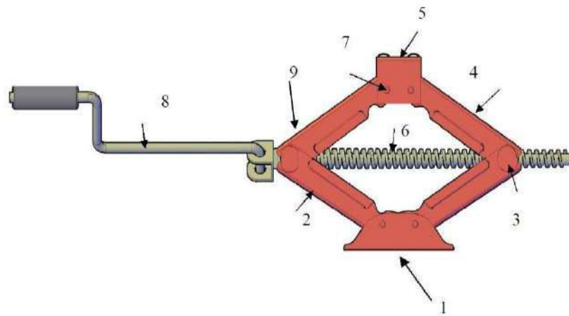
Gambar 2.3 Komponen-komponen Dongkrak Ulir Mekanis
