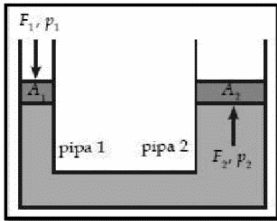
Gambar 2.7 gambar tekanan F1 di pipa satu sama besar dengan gaya angkat di pipa dua
