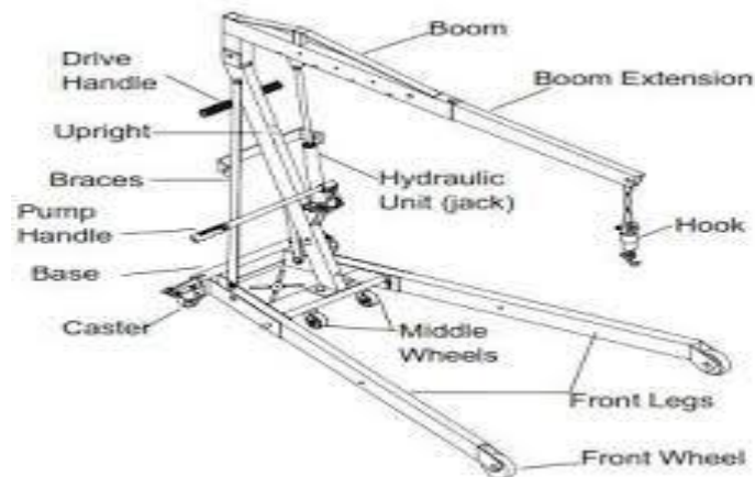
Gambar 2.1 Konstruksi Elektrik Crane
