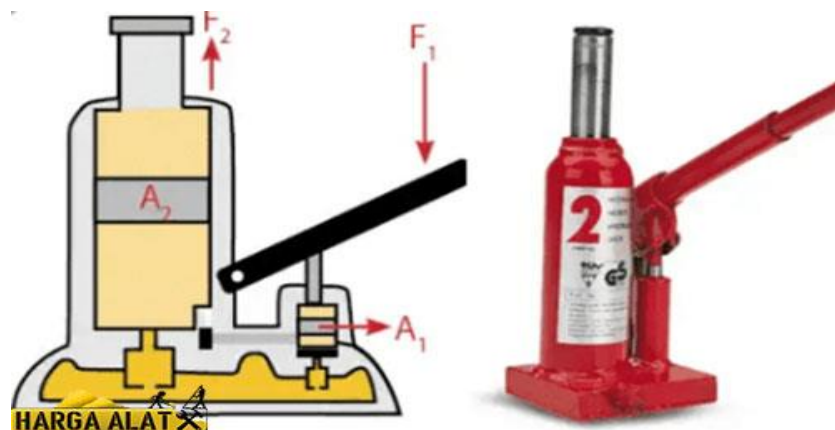
Gambar 2.5 Cara Kerja Dongkrak Hidrolik
