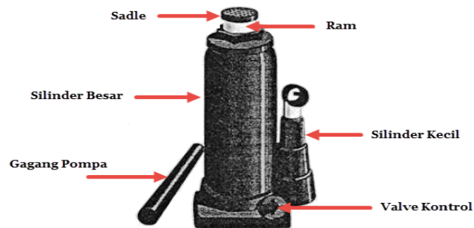
Gambar 2.4 Komponen Dongkrak Hidrolik
