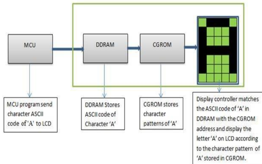
Gambar 2.16 Proses Terbentuknya Karakter Pada Dot Matrik 5 x 7 LCD (Sumber: http://www.npeducations.com/2012/08/custom-character-generation-on-16x2-lcd.html )
