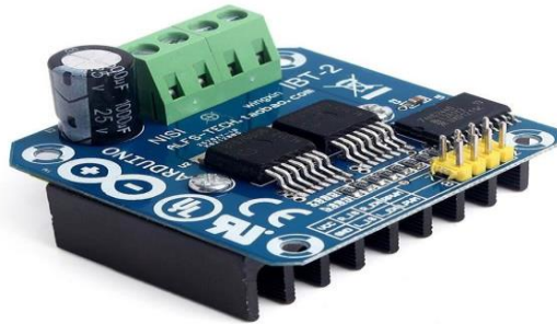
Gambar 2.7 Bentuk Motor Driver
