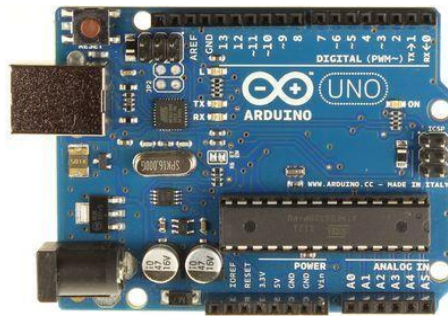
Gambar 2.6 Arduino UNO R3
