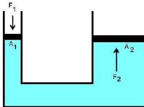
Gambar 2.3 Prinsip Hukum Pascal
