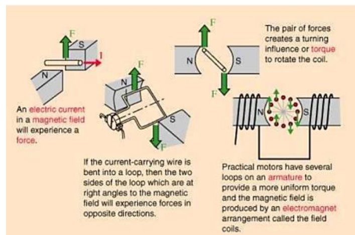
Gambar 2.9 Prinsip Dasar Kerja Motor Listrik (Sumber: https://zoniaelektro.net/motor-listrik/ )
