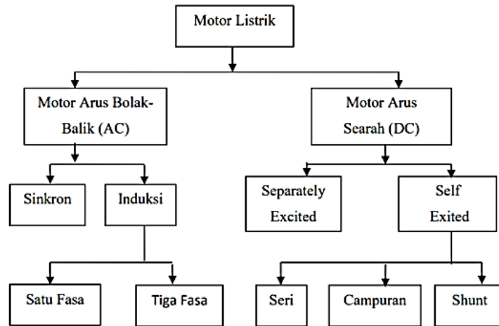
Gambar 2.10 Klasifikasi Motor Listrik.
