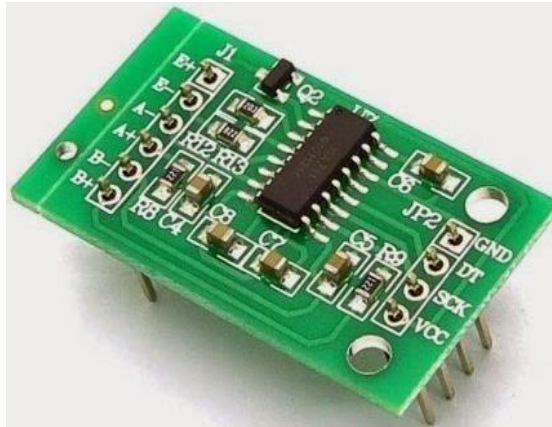
Gambar 2.5 Modul Penguat HX711
