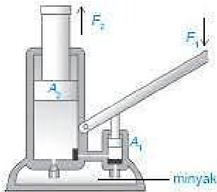
Gambar 2.2 Dongkrak Tabung Hidrolik (Sumber: Prihatin JY dkk, 2018)
