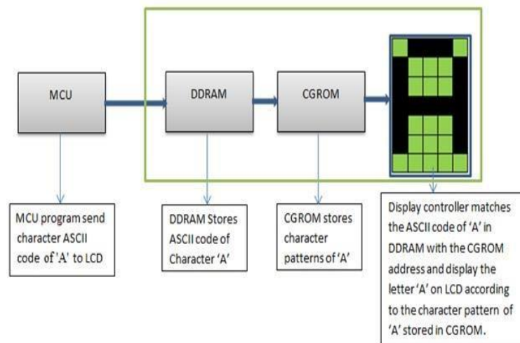
Gambar 2.17 Proses Terbentuknya Karakter Pada Dot Matrik 5 x 7 LCD (Sumber: Google)
