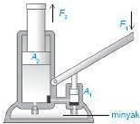
Gambar 2.1 Dongkrak Tabung Hidrolik (Sumber: Google)
