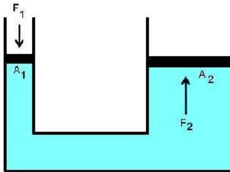
Gambar 2.2 Prinsip Hukum Pascal (Sumber: Google)
