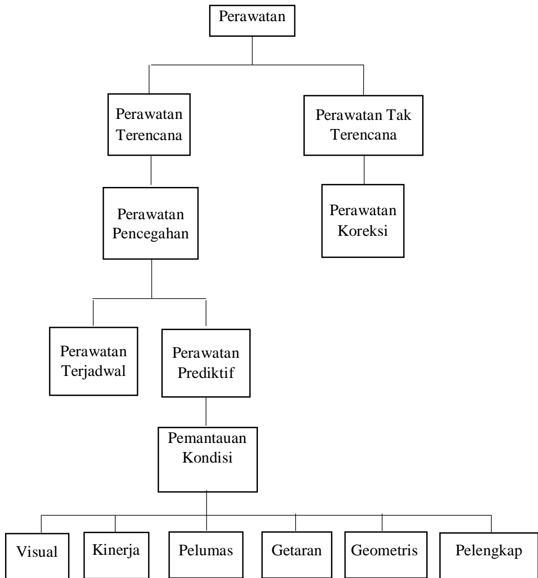
Gambar 2.18 Bagan Perawatan dan Perbaikan (Sumber: Google)
