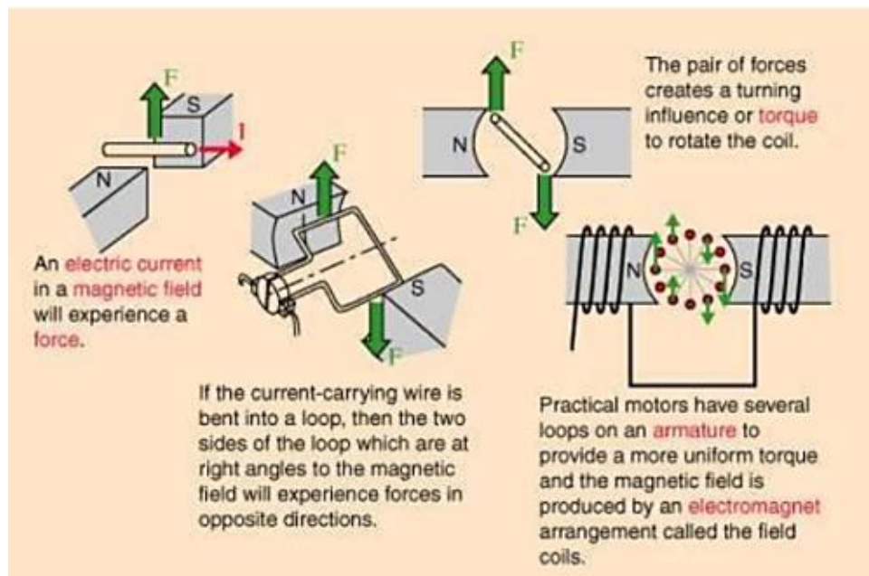
Gambar 2.10 Prinsip Dasar Kerja Motor Listrik
