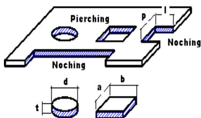
Gambar 2.30 jenis potong
