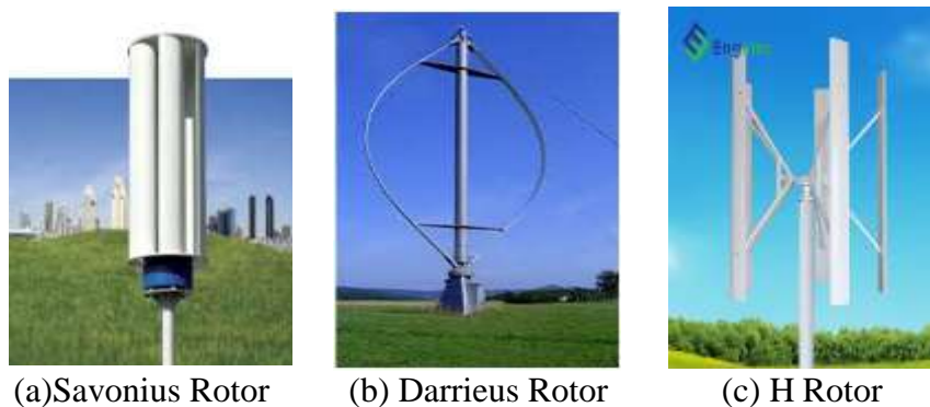
Gambar 2.5 Turbin Angin Sumbu Vertikal 16
