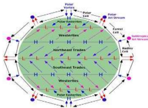
Gambar 2.1 Pola Sirkulasi Udara Akibat Rotasi Bumi 18
