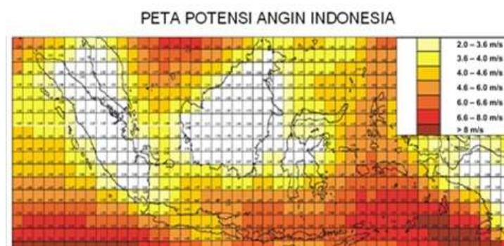
Gambar 2.2 Peta Potensi Angin Indonesia 7
