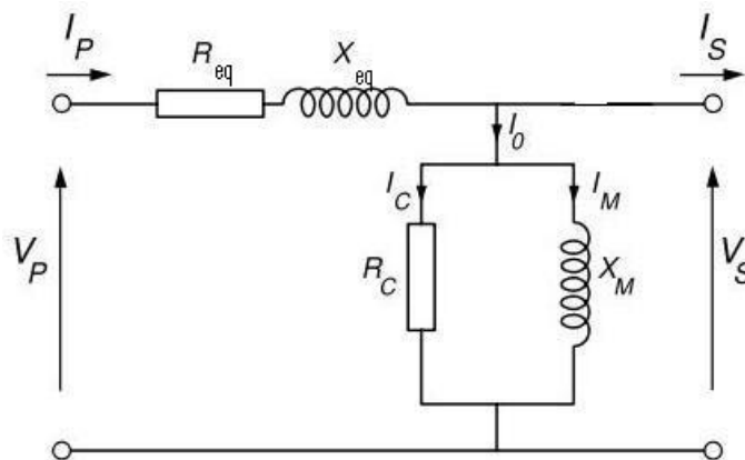
Gambar 2.5 Rangkaian Ekuivalen Transformator
