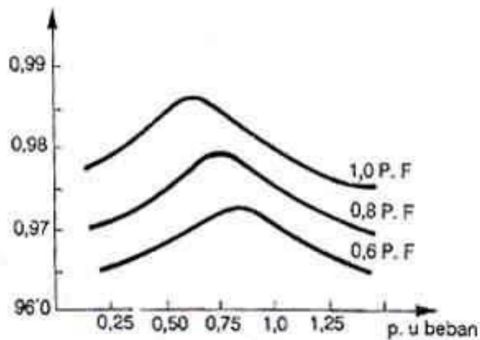
Gambar 2.18 Hubungan antara efisiensi dengan beban pada \cos\Phi yang berbeda-beda 5
