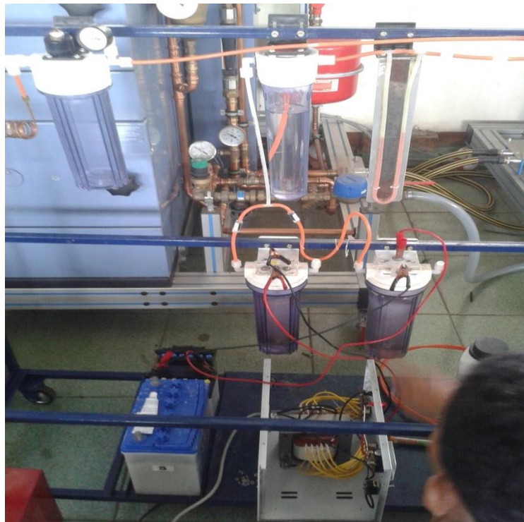
Gambar 27. Merangkai Kabel Supplay Arus Listrik dari Batre ke Reaktor Elektrolisis
