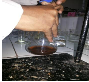
(d) Titrasi
