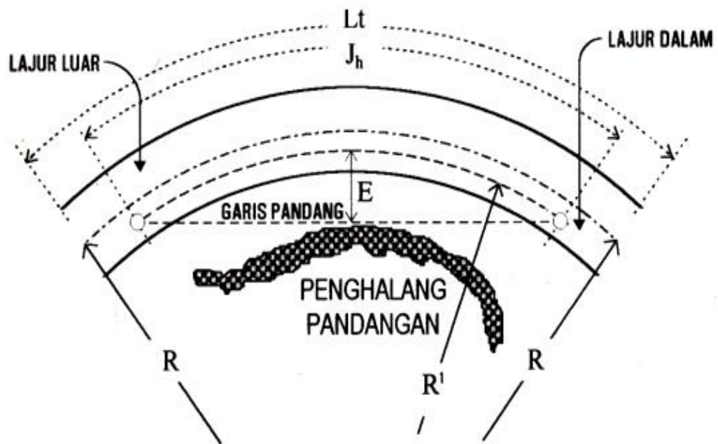
Gambar 2.11 Daerah bebas samping ditikungan untuk J_h < L_t
