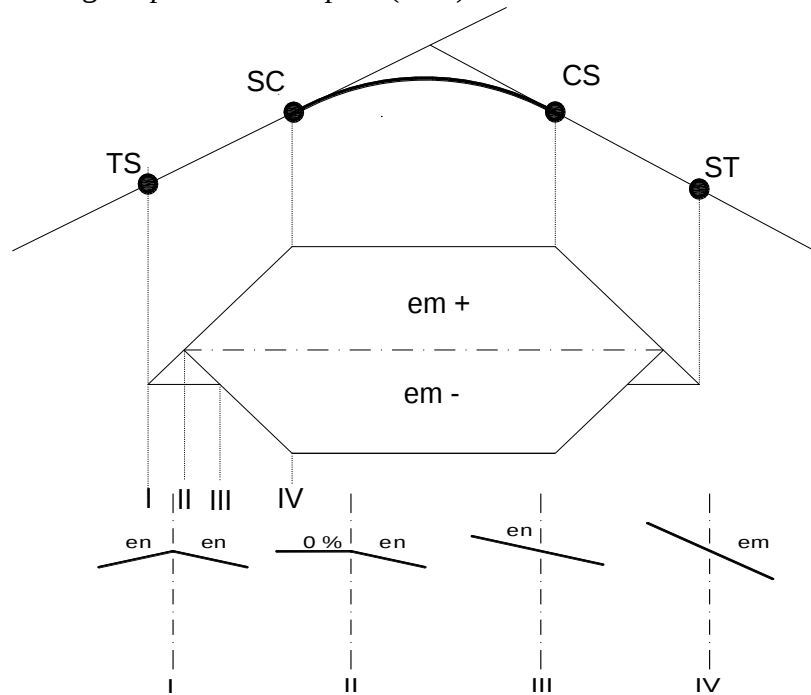
Gambar 2.8 Pencapaian Superelevasi Tikungan Spiral-Circle-Spiral
