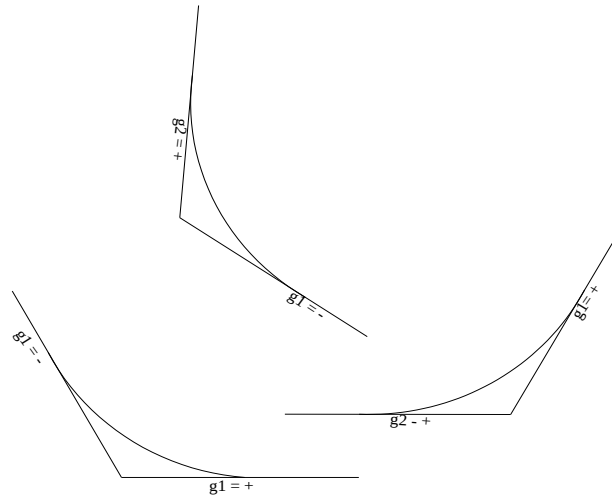
Gambar 2.17 Alinyemen Vertikal Cekung
