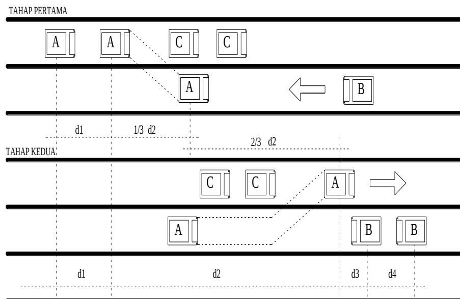
Gambar 2.10 Jarak Pandang Mendahului
