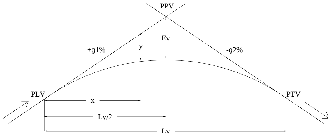
Gambar 2.13 Lengkung Vertikal
