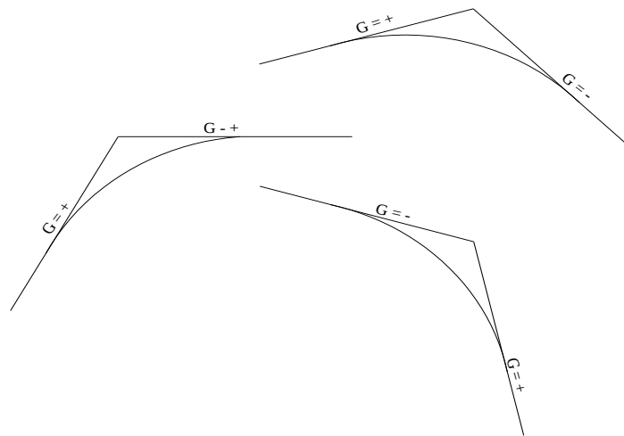
Gambar 2.14 Alinyemen Vertikal Cembung
