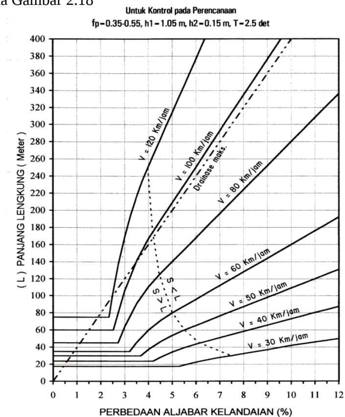
Gambar 2.18 Grafik Panjang Lengkung Vertikal Cekung
