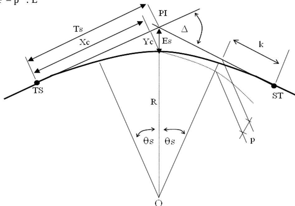
Gambar 2.6 Tikungan SpiralSpiral
