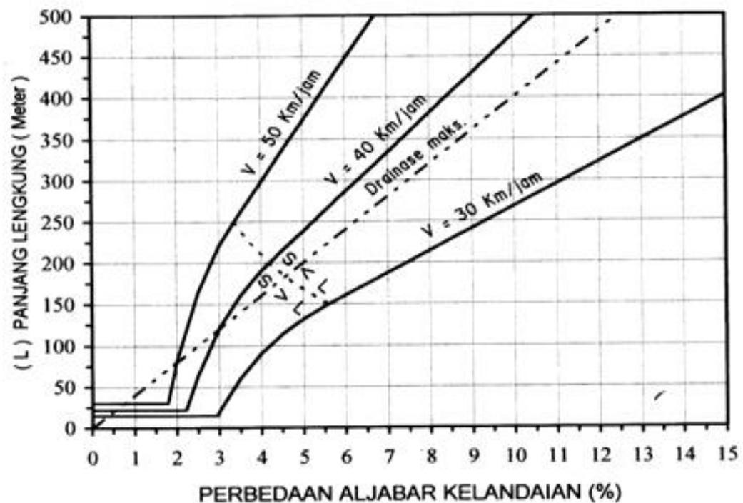
Gambar 2.16 Grafik Panjang Lengkung Vertikal Cembung berdasarkan Jarak Pandang Mendahului ( J_d )
