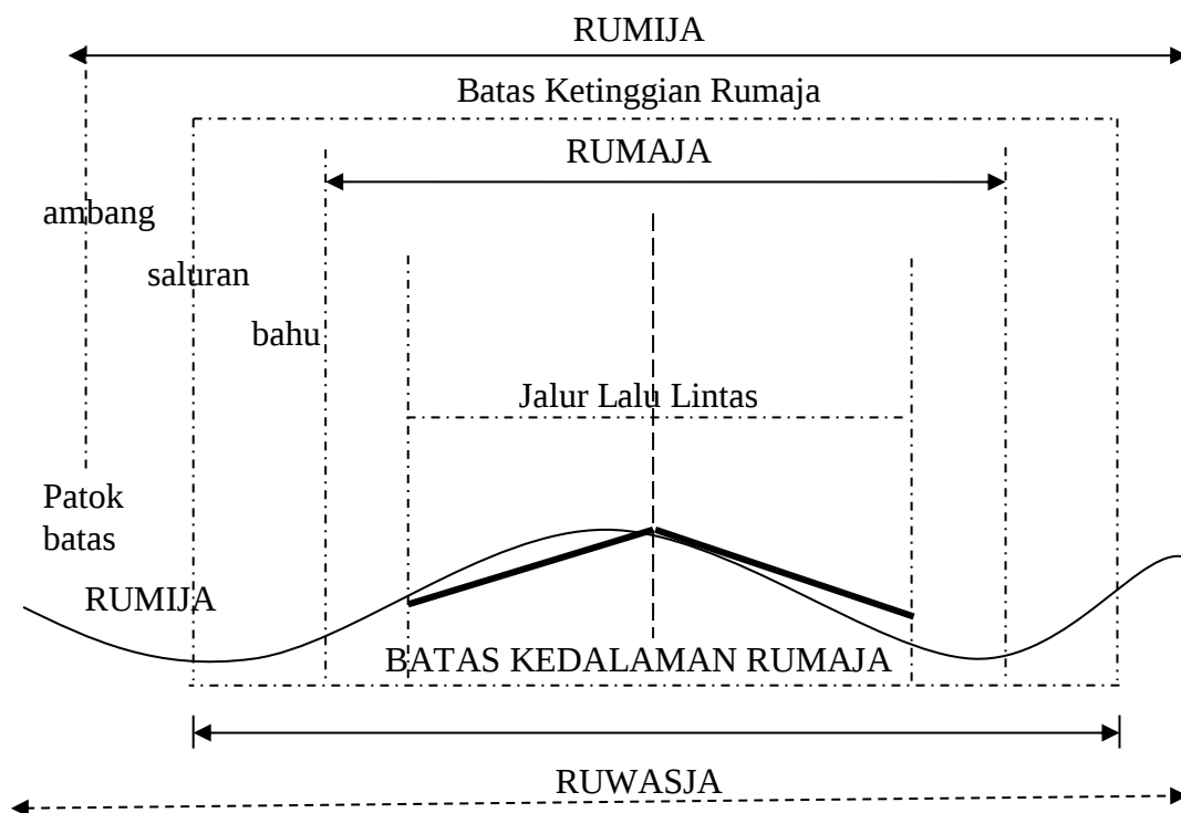
Gambar 2.3 Rumaja, Rumija, Ruwasja di Lingkungan jalan antar kota.
