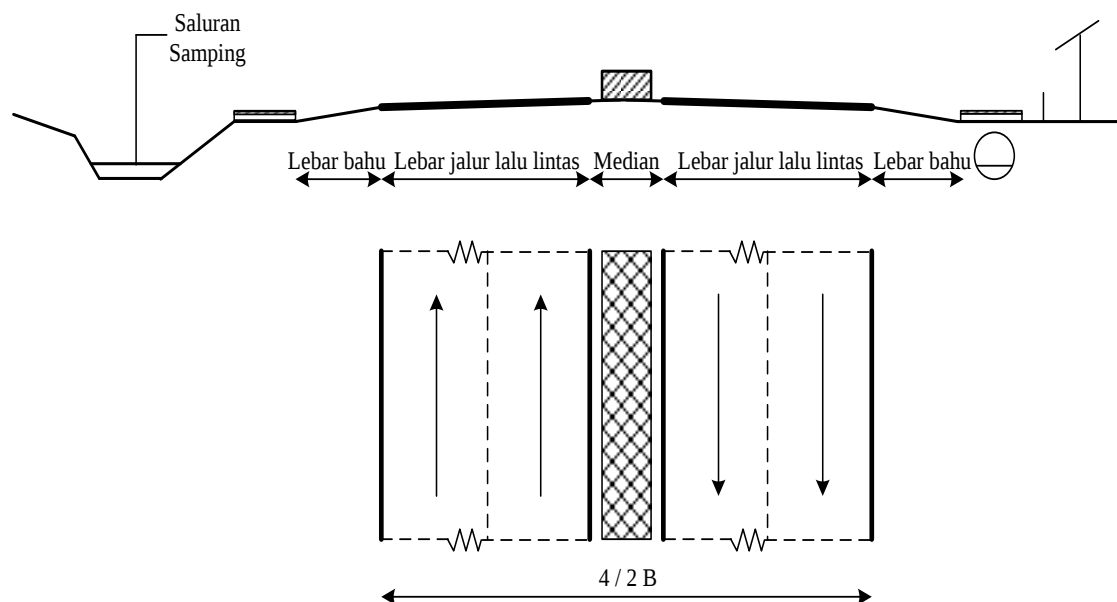
Gambar 2.2 Tipikal Potongan Melintang Normal dan Denah Untuk 4 / 2 B
