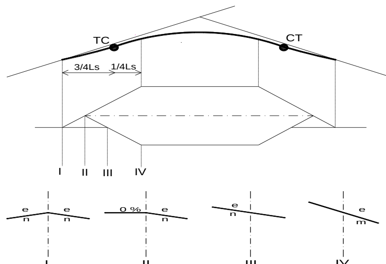
Gambar 2.7 Pencapaian Superelevasi Tikungan Full Circle
