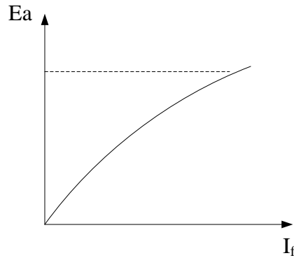
Gambar 2.6 Grafik Hubungan Arus Penguat Medan ( I_f ) dan E_a 7
