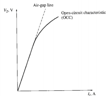
Gambar 2.10 Karakteristik Open Circuit pada Generator 5
