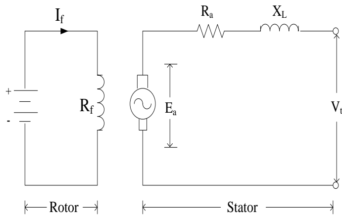
Gambar 2.5 Rangkaian Ekuivalen Generator Sinkron Tanpa Beban 9
