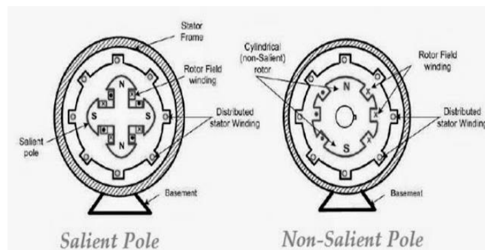
Gambar 2.4 Rotor Bentuk Menonjol dan Bentuk Silinder 12
