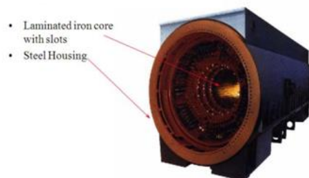
Gambar 2.3 Konstruksi Stator 5
