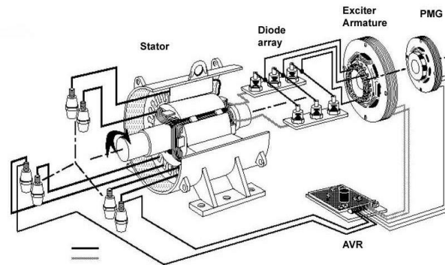
Gambar 2.16 Rotor, kumparan AC exciter , rotating diode dan PMG yang terletak satu poros 14
