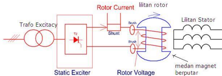
Gambar 2.13 Sistem Eksitasi dengan Sikat ( Brush Excitation ) 13
