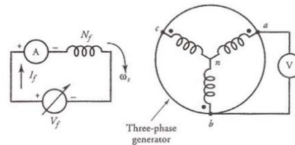
Gambar 2.9 Diagram Rangkaian Tes Open Circuit 5
