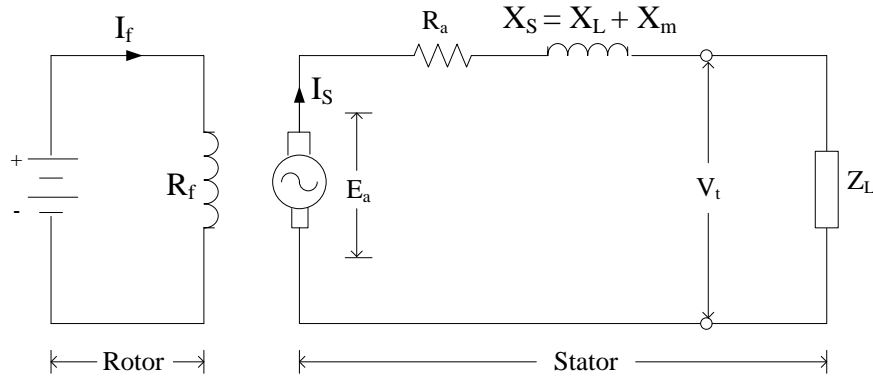
Gambar 2.7 Rangkaian Ekuivalen Generator Sinkron Berbeban 9
