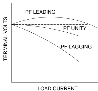
Gambar 2.8 Karakteristik Generator AC Pada Berbagai Faktor Daya 9
