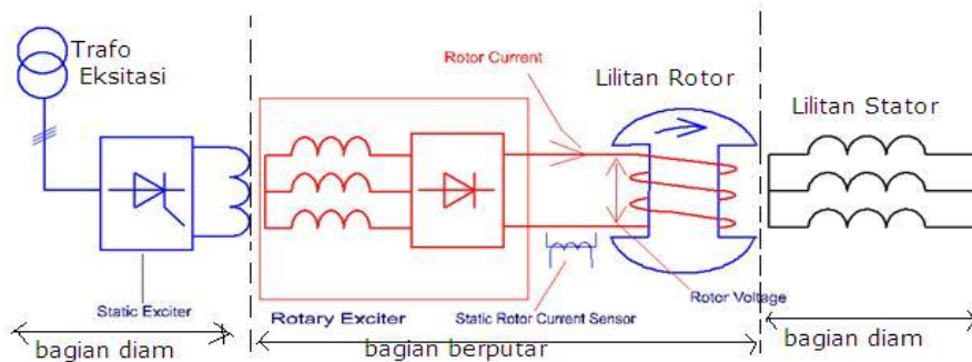
Gambar 2.14 Sistem Eksitasi Tanpa Sikat ( Brushless Excitation ) 13
