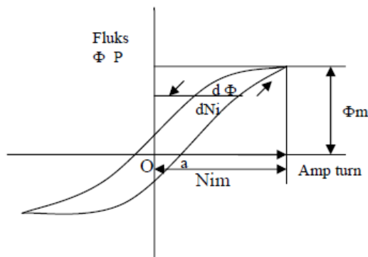
Gambar 2.21 Lingkaran Histerisis
