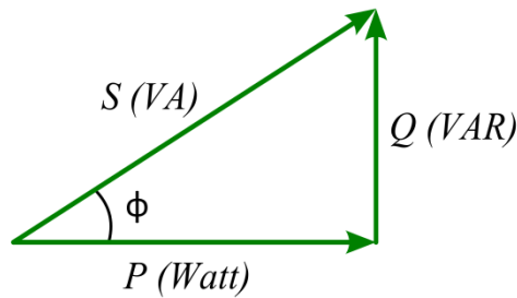
Gambar 2.9. Segitiga daya
