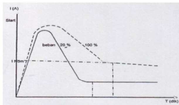
Gambar. 2.6. Karakteristik start
