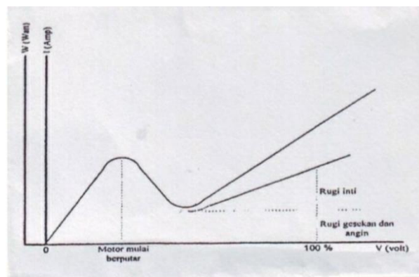
Gambar 2.4. Karakteristik Beban Nol
