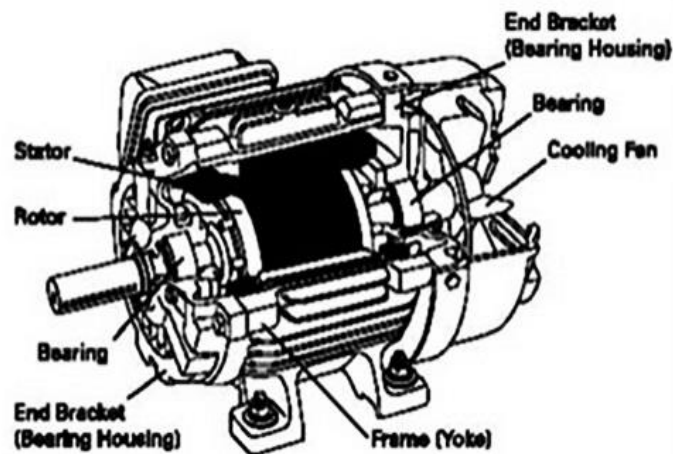
Gambar 2.1. Fisik Motor Induksi
