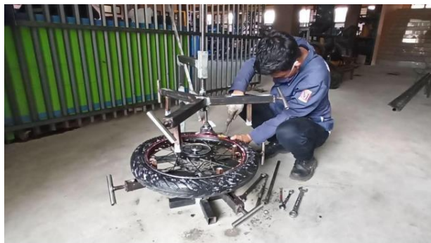
Gambar 5.5 Proses Setting Posisi Ban (Sumber; Dokumentasi)
