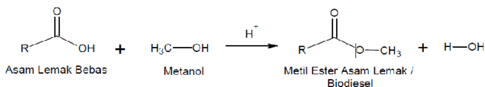
Gambar 1. Reaksi Esterifikasi
