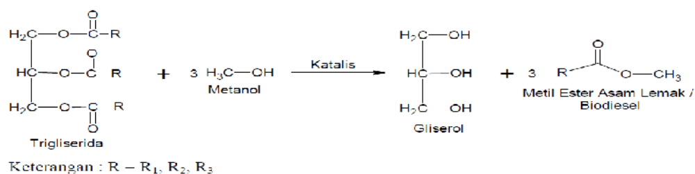
Gambar 2. Reaksi Transesterifikasi
